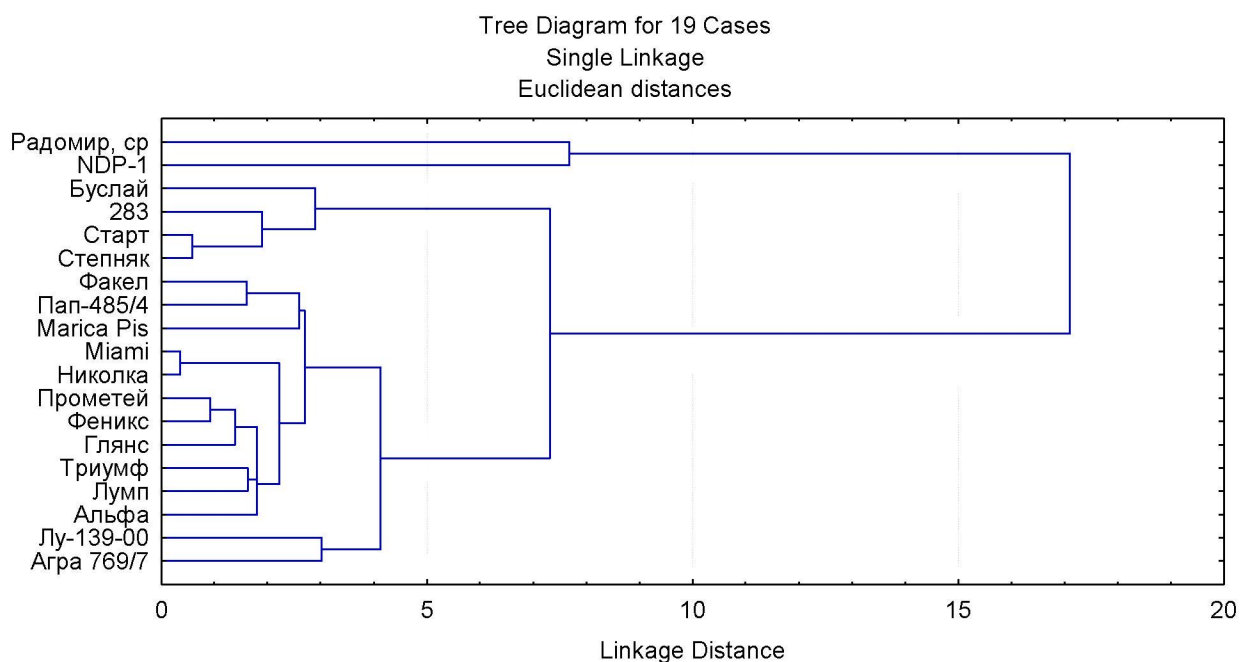
Рисунок 2. Дендрограмма распределения образцов гороха на кластеры по высоте растений и их устойчивости к полеганию (2021 – 2023 гг.) (Эвклидово расстояние между точками)
