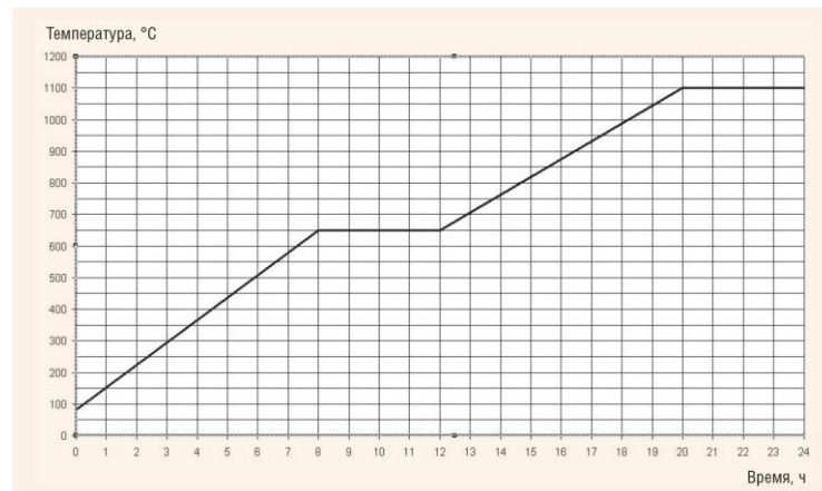
Рисунок 1 – Температурный график
