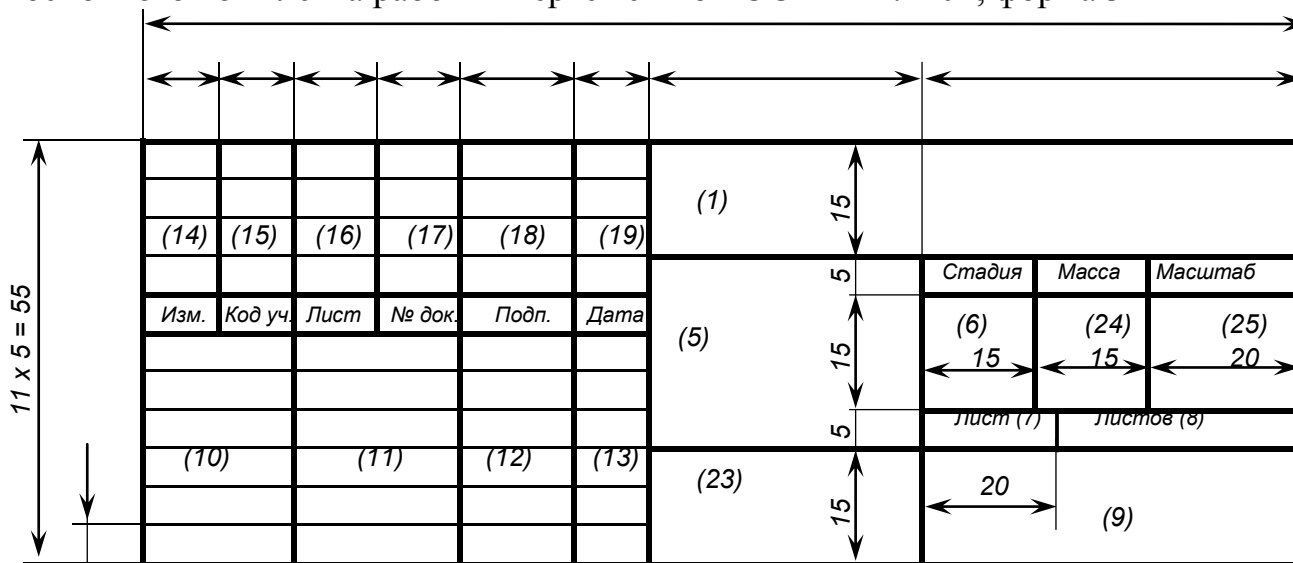
Рисунок С.4 – Основная надпись и дополнительные графы к ней на листах основного комплекта рабочих чертежей по ГОСТ Р 21.1101, форма 3
