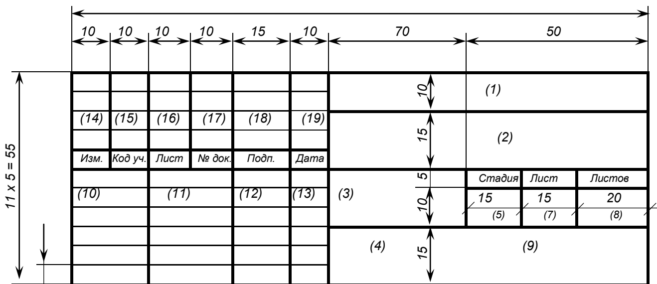
Рисунок С.3 – Основная надпись для чертежей (схем) и текстовых конструкторских документов (последующие листы) по ГОСТ 2.104, форма 2а 185
