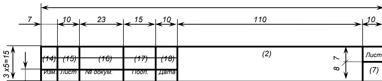
Рисунок С.3 – Основная надпись для чертежей (схем) и текстовых конструкторских документов (последующие листы) по ГОСТ 2.104, форма 2а 185
